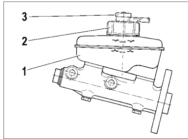
Рис. 35. Бачок гидропривода тормозов
